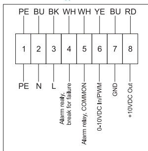
Схема подключения № 2
