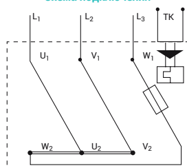
Схема подключения
