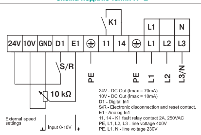
Схема подключения № 2
