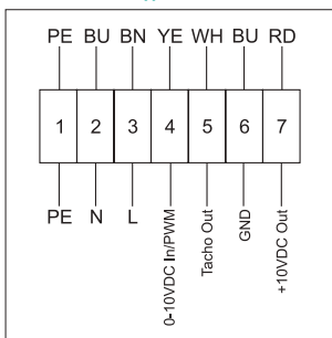
Схема подключения № 1
