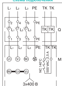
Схема подключения
