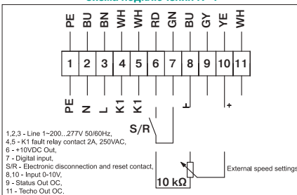
Схема подключения № 1
